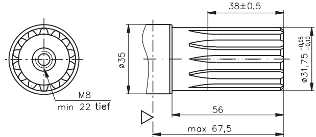
HB - \varnothing 1\frac{1}{4} " vielkeilwelle 14T, DP12/24 ANSI B92.1-1976 Max. Drehmomentabgabe 77 daNm
