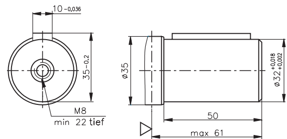
CB - \varnothing 32 zylindrisch, Paßfeder A10x8x40 DIN 6885 Max. Drehmomentabgabe 77 daNm
