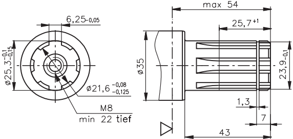
SH - vielkeilwelle, BS 2059 (SAE 6B) Max. Drehmomentabgabe 44 daNm
