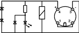
Schaltbild:
